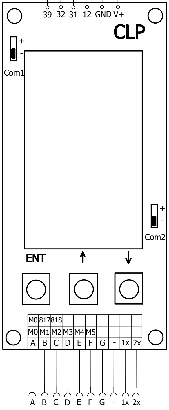
Kumanda Panosu 7-Segment Çıkışları
