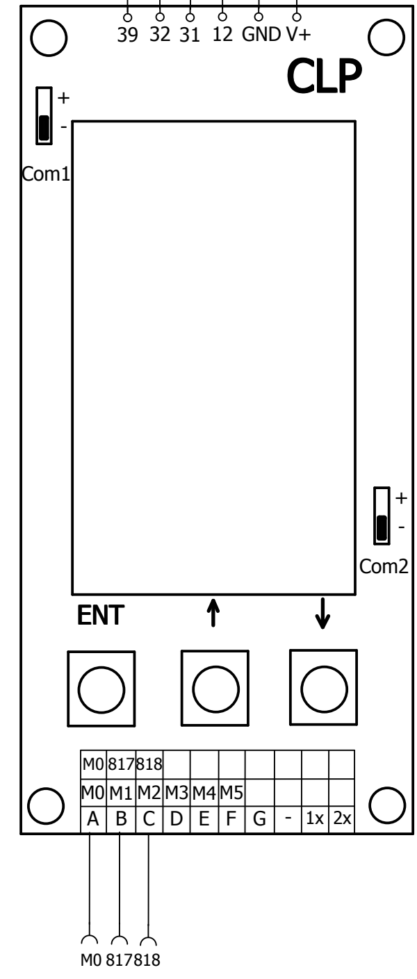
Kumanda Panosu Sayıcı ve Limit Şalter Çıkışları
