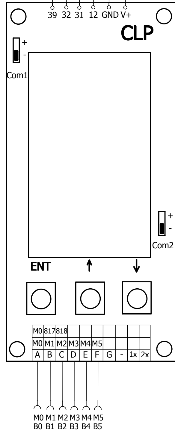
Kumanda Panosu Gray/Binary Kod Çıkışları
