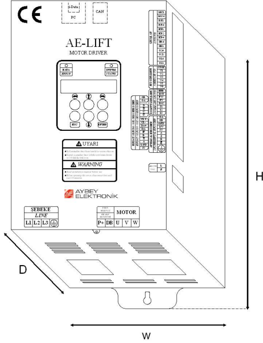
Şekil 2.1 Sürücü Kutusu
