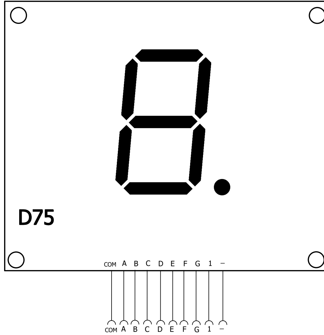
Kontrol Panolsu 7 Segment Çıkışları
