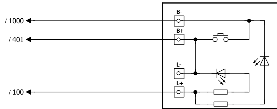
ÇİFT RENK TWO COLOR KAYIT BUTONU CALL BUTTON
